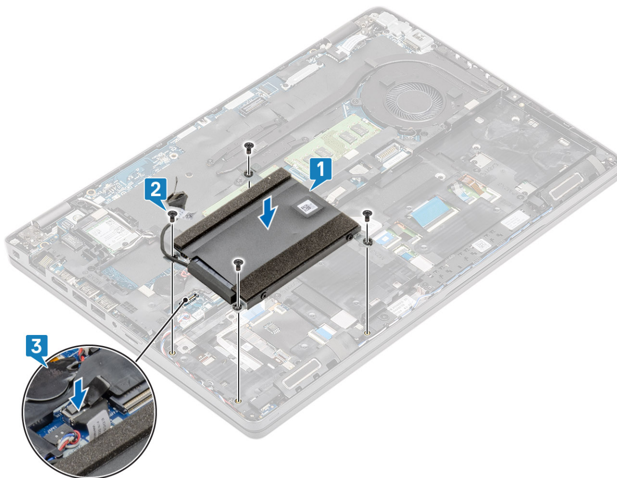
Obrázek 4. Montáž jednotky pevného disku
