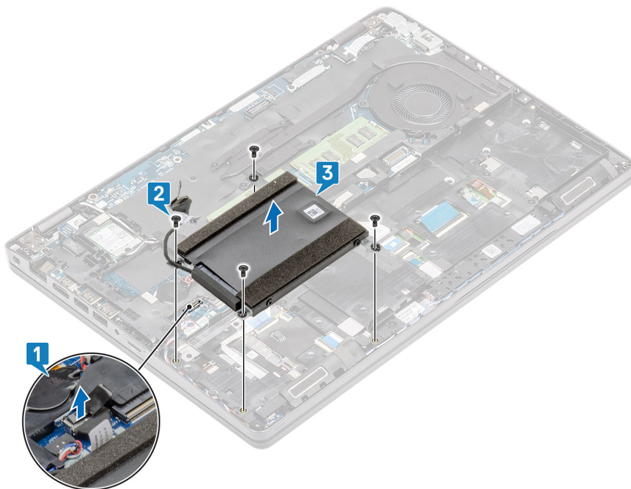
Obrázek 3. Demontáž jednotky pevného disku
